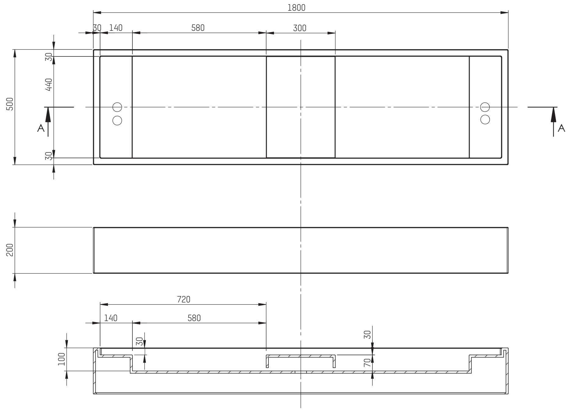
SECTION A-A
