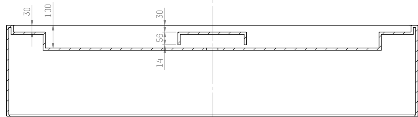
SECTION A-A
