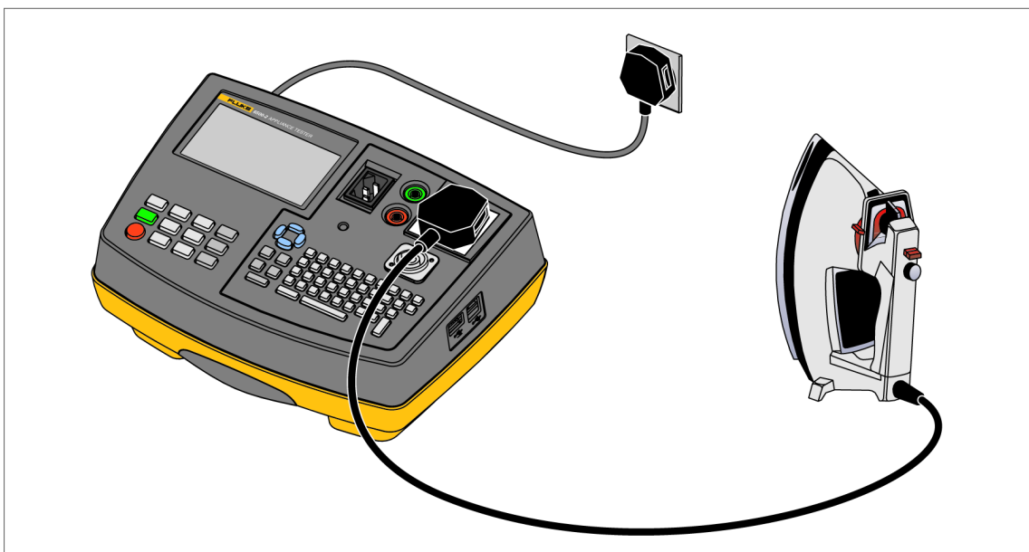
Afbeelding 8. Aansluitingen voor belastings-/lekstroomtest
