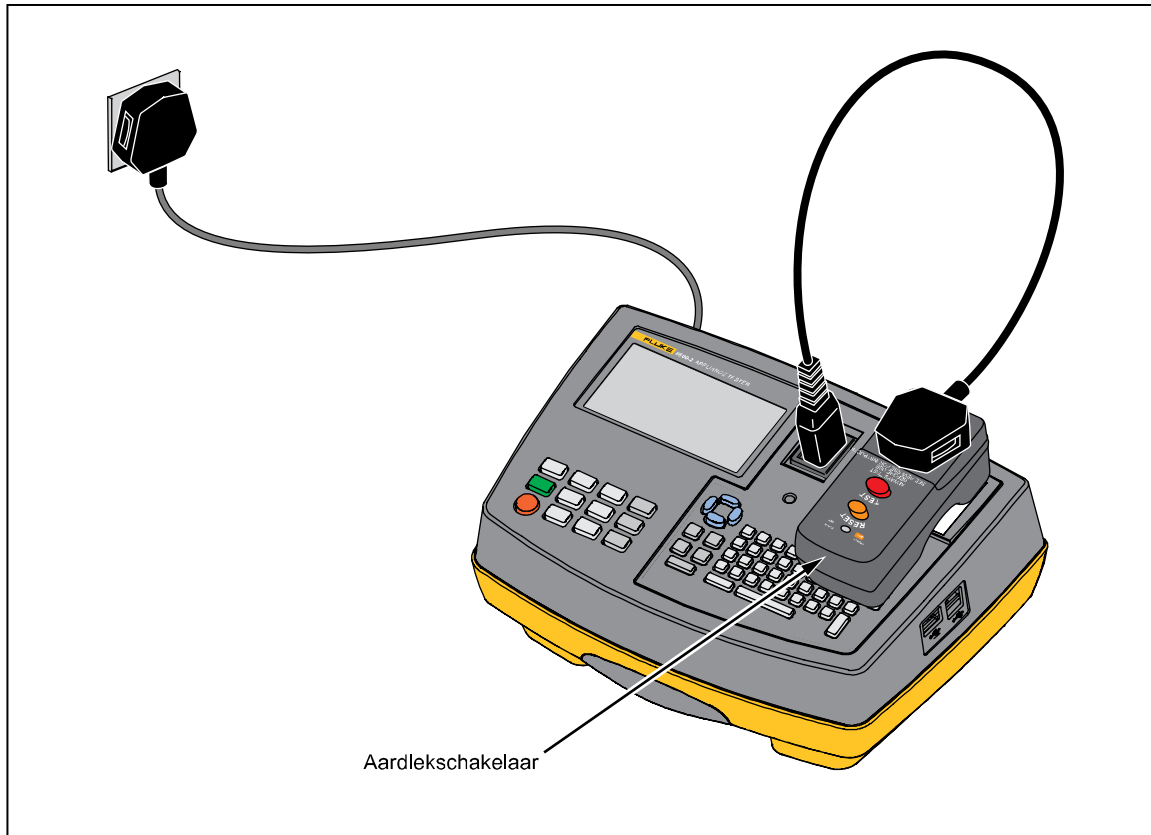
Afbeelding 9. Testen van universele AC-aardleischakelaars
