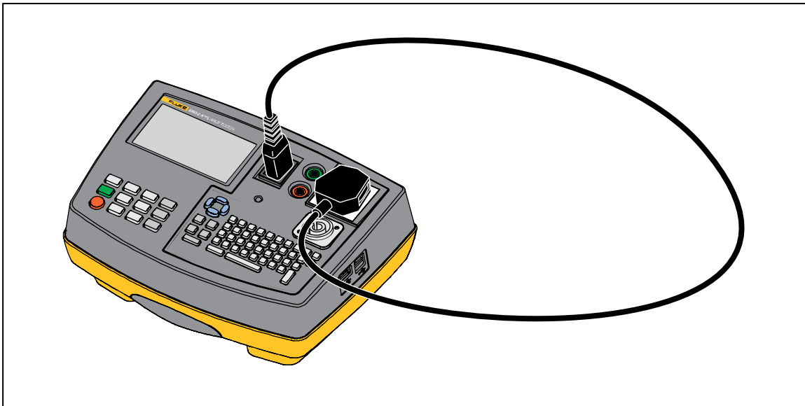
Afbeelding 10. Aansluiting voor IEC-apparatensnoertest
