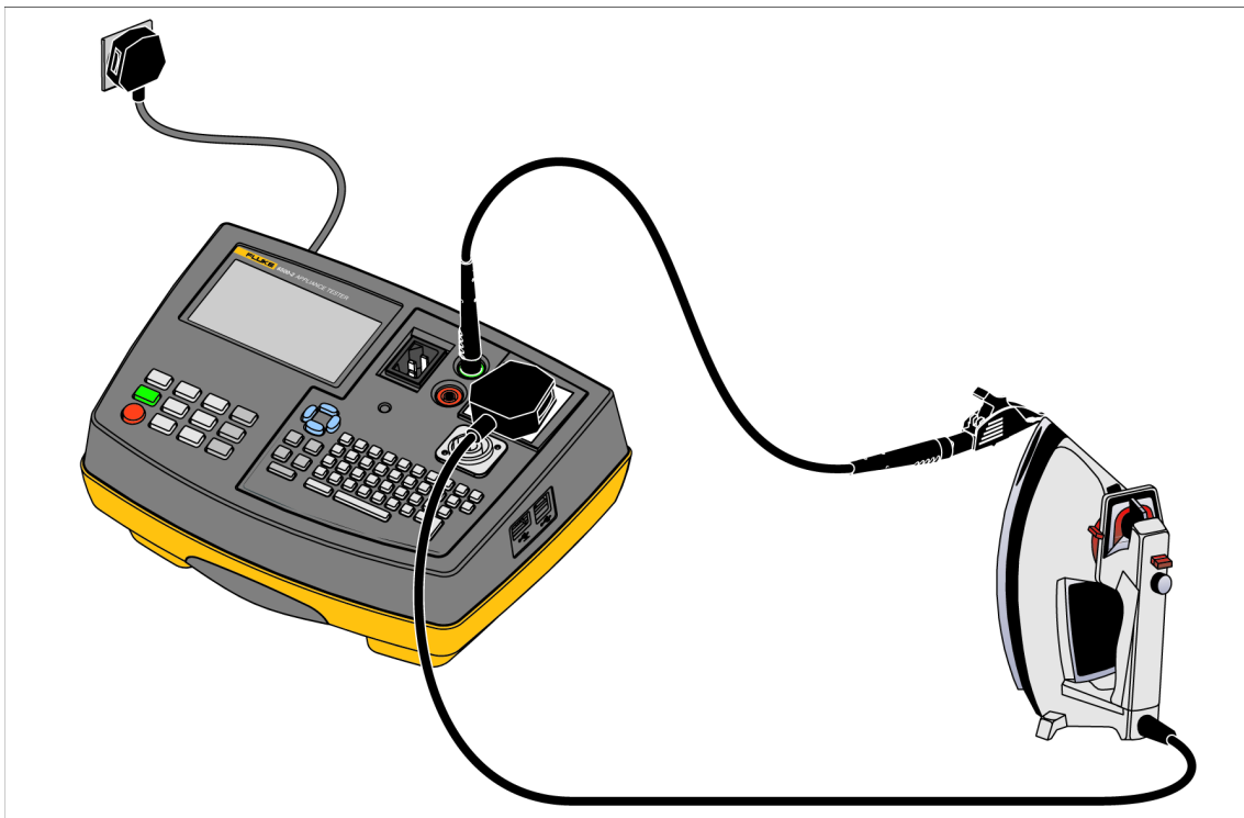
Afbeelding 2. Beschermingsleidingtest
