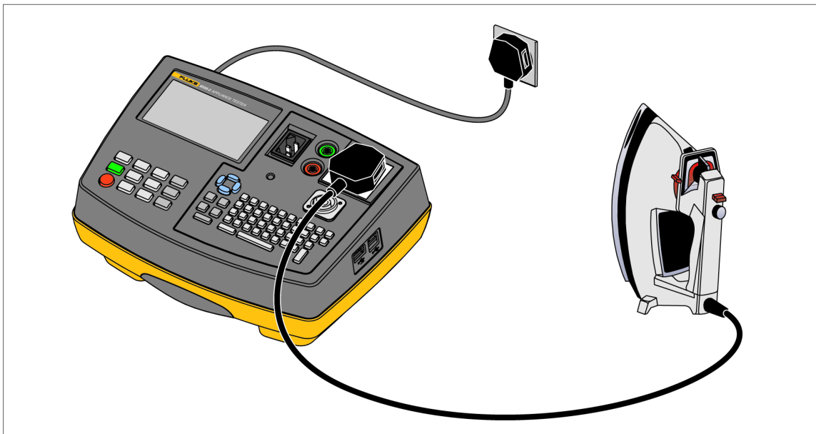
Afbeelding 3. Aansluitingen voor isolatietest voor klasse 1
