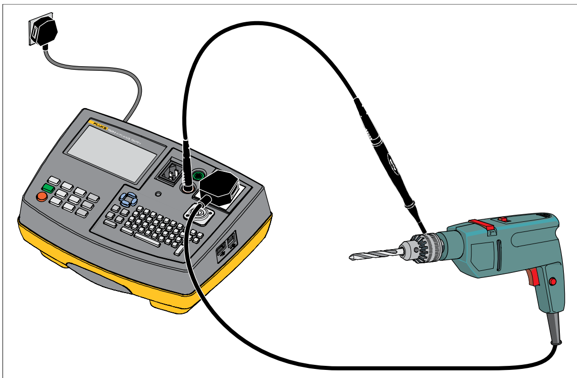
Afbeelding 4. Aansluitingen voor isolatietest voor klasse II
