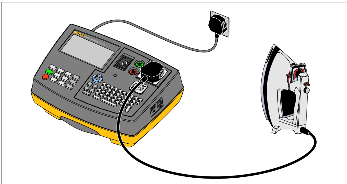
Afbeelding 5. Aansluitingen voor vervangende-lekstroomtest voor klasse I
