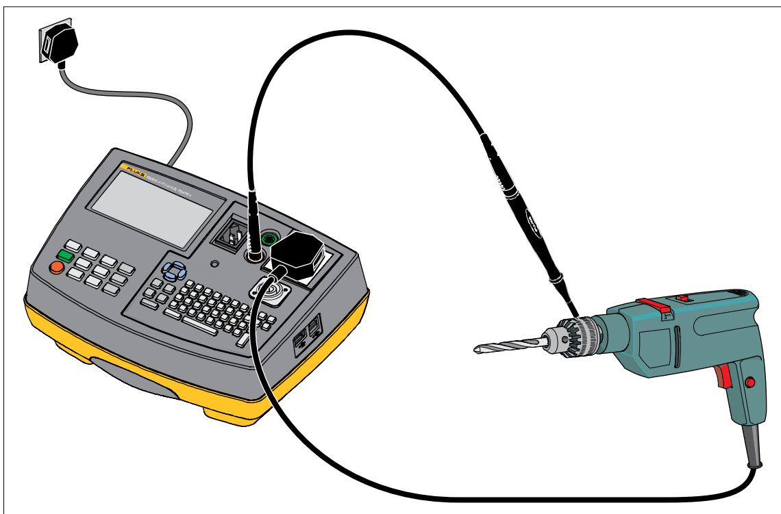
Afbeelding 6. Aansluitingen voor vervangende-lekstroomtest voor klasse II
